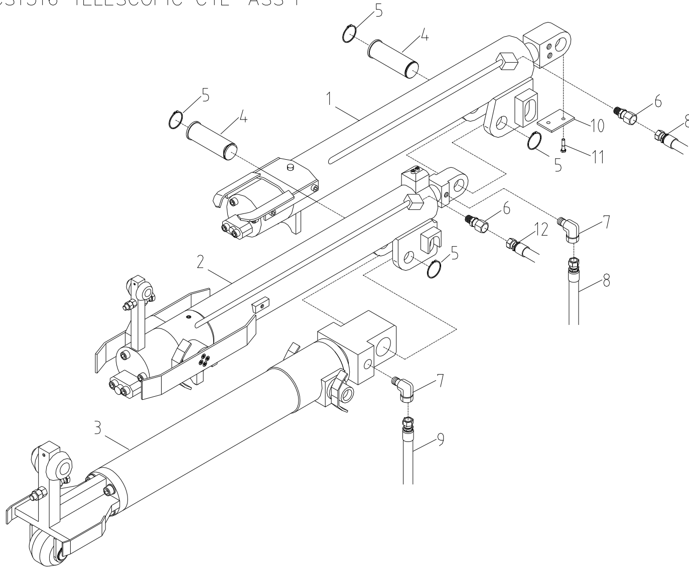
텔레스코픽 실린더 조립체 Fig. 1-1 SCS1516 TELESCOPIC CYL' ASS'Y
