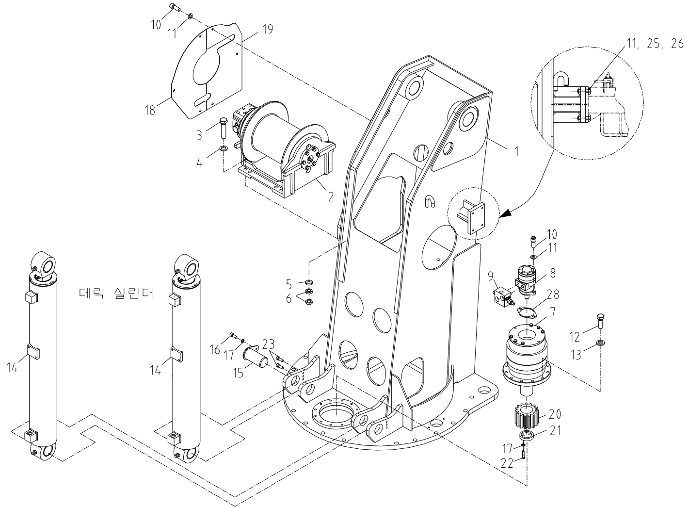
스윙 포스트 조립체 Fig. 2 SCS1516 SWING POST ASS'Y
