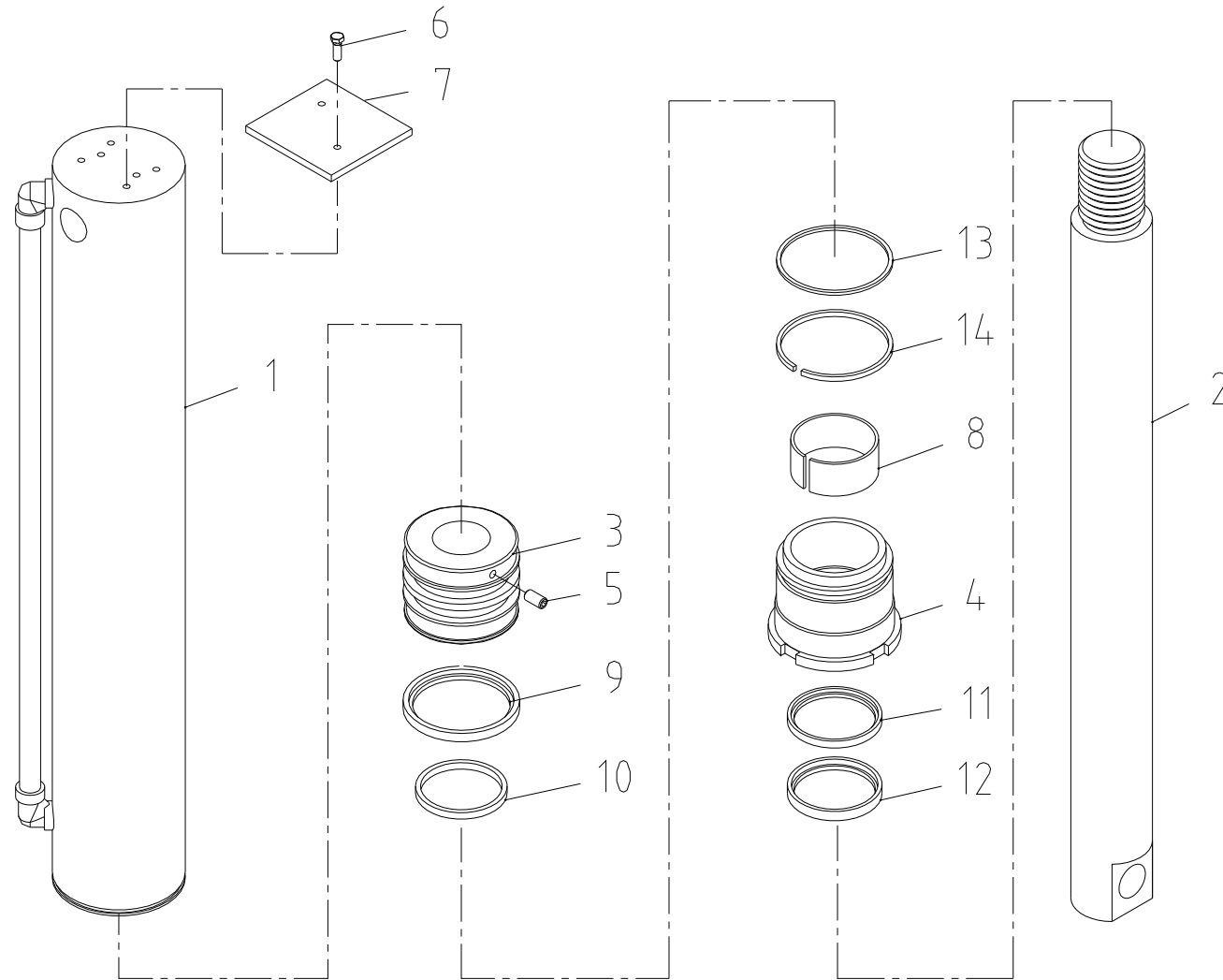
잭 실린더 조립체 Fig. 9-2-1-1 SCS1516 JACK CYL' ASS'Y
