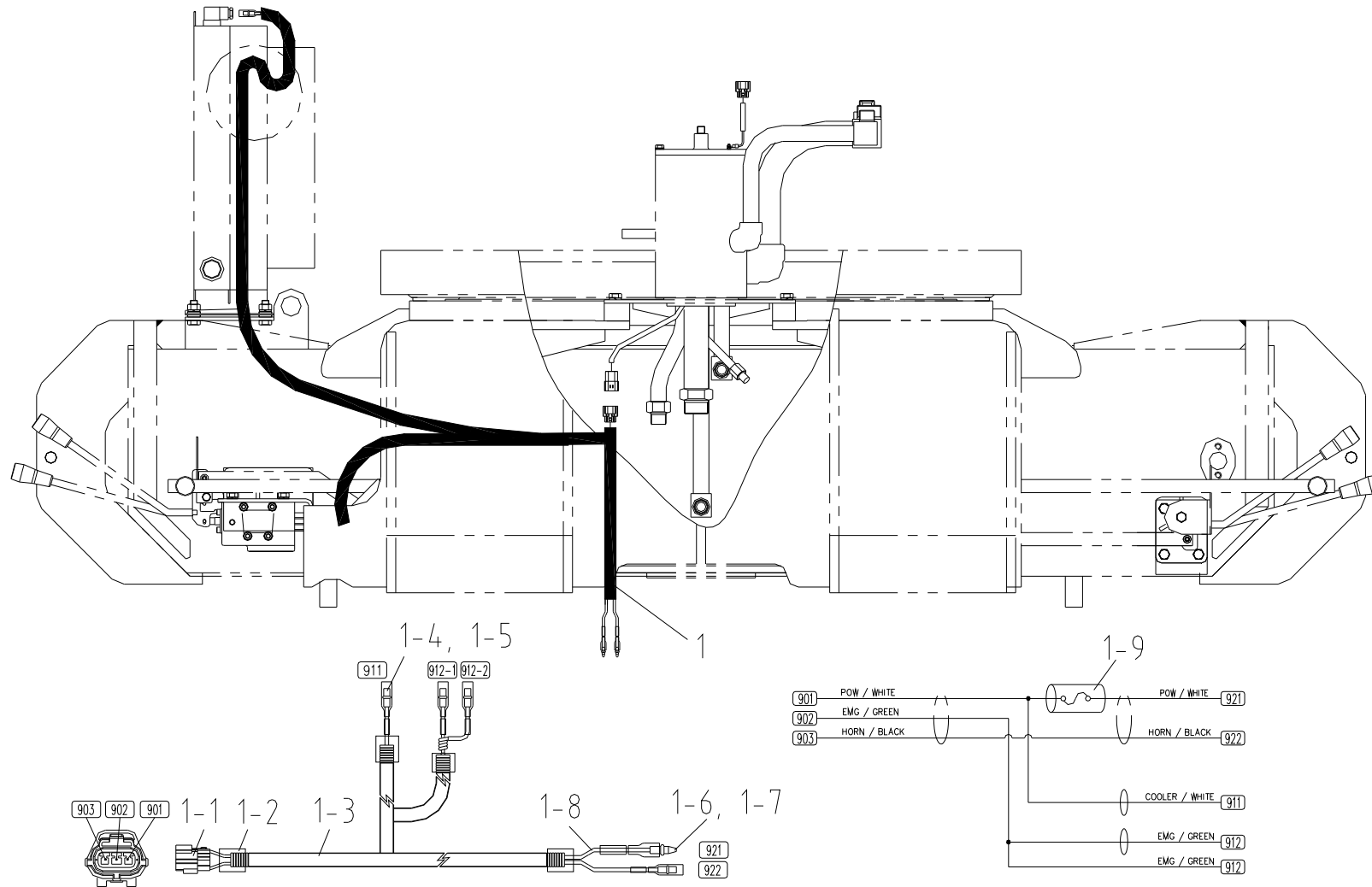
프레임 전선 Fig. 10-1 SCS1516 FRAME WIRING
