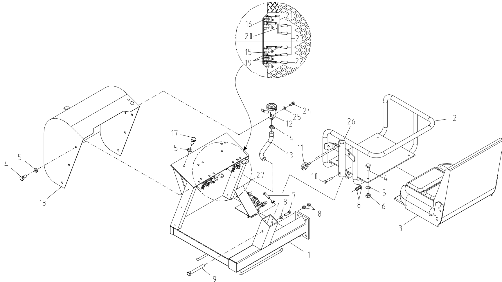
탑 시트 조립체 Fig. 6 SCS1516 TOP SEAT ASS'Y
