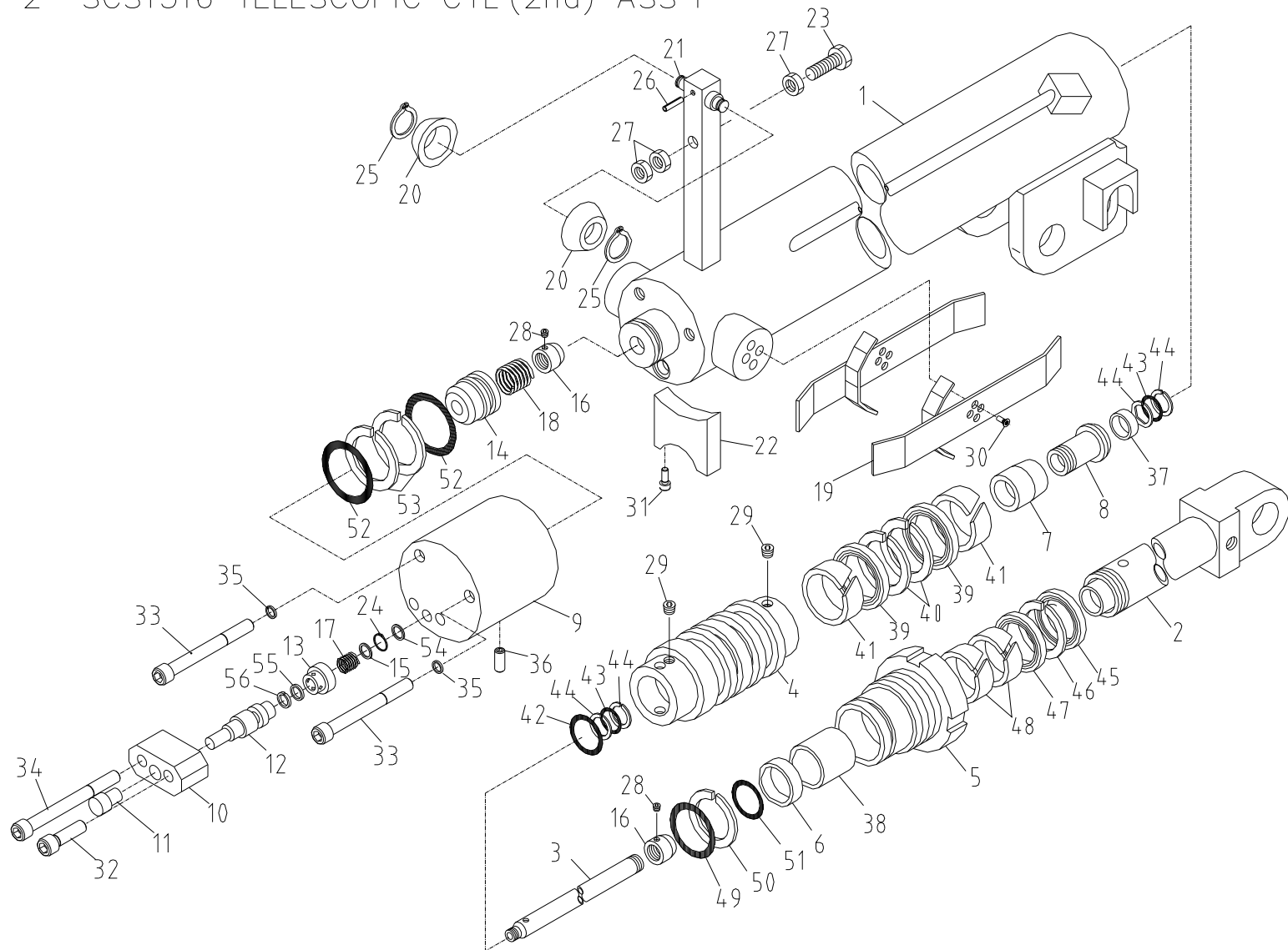
텔레스코픽 실린더(2단) 조립체 Fig. 1-1-2 SCS1516 TELESCOPIC CYL'(2nd) ASS'Y
