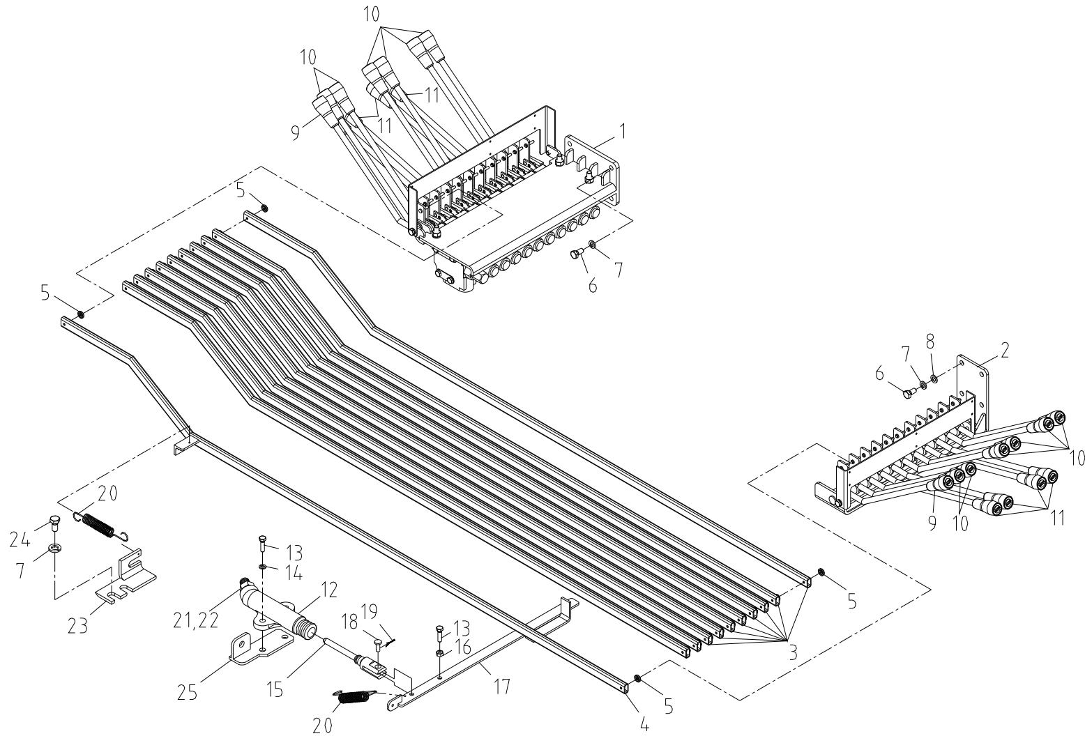
오퍼레이션 조립체 Fig. 3-2 SCS1516 OPERATION ASS'Y
