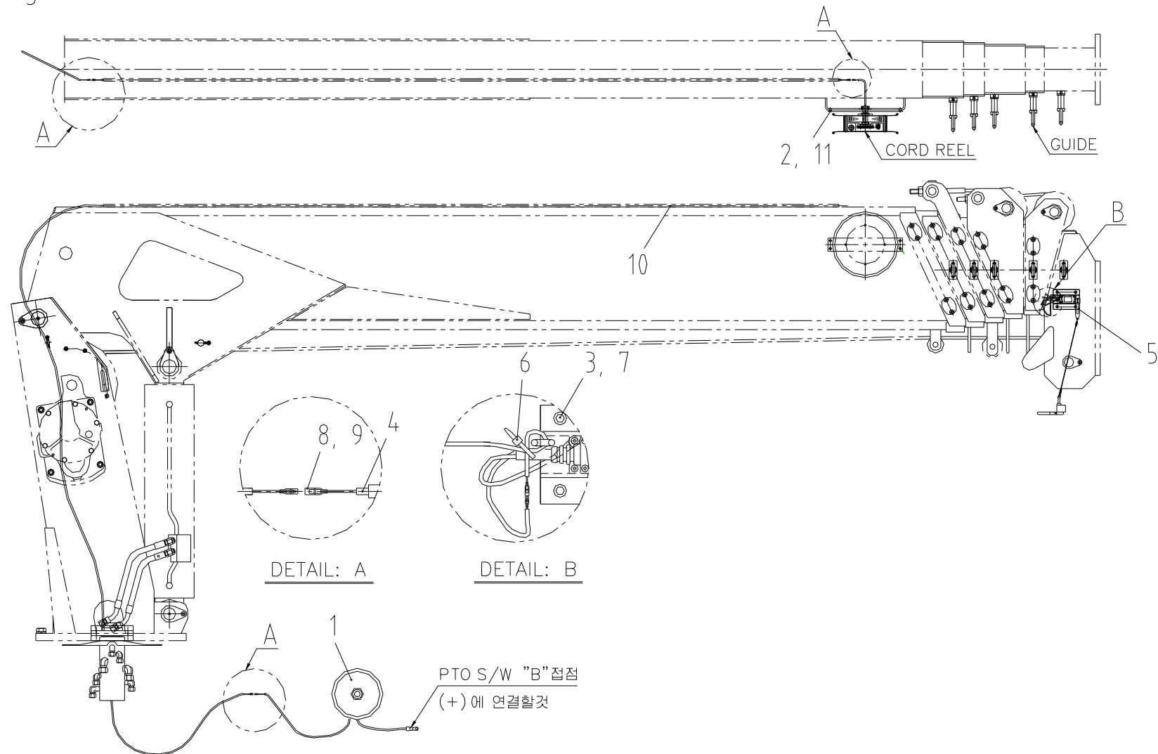
Fig. 15 과권방지장치 조립체
