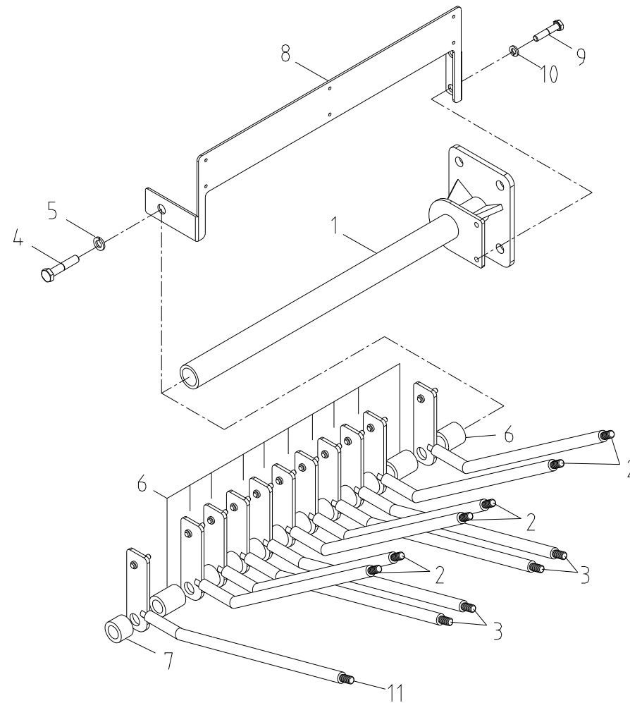
레버 스텐드 셋 Fig. 3-2-2 SCS1516 LEVER STAND SET
